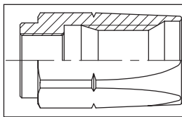
2000-01 ОБЖИМНАЯ ВТУЛКА R1 Рукав без снятия оболочки
