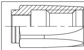
2000-03 ОБЖИМНАЯ ВТУЛКА R1 AT Рукав без снятия оболочки
